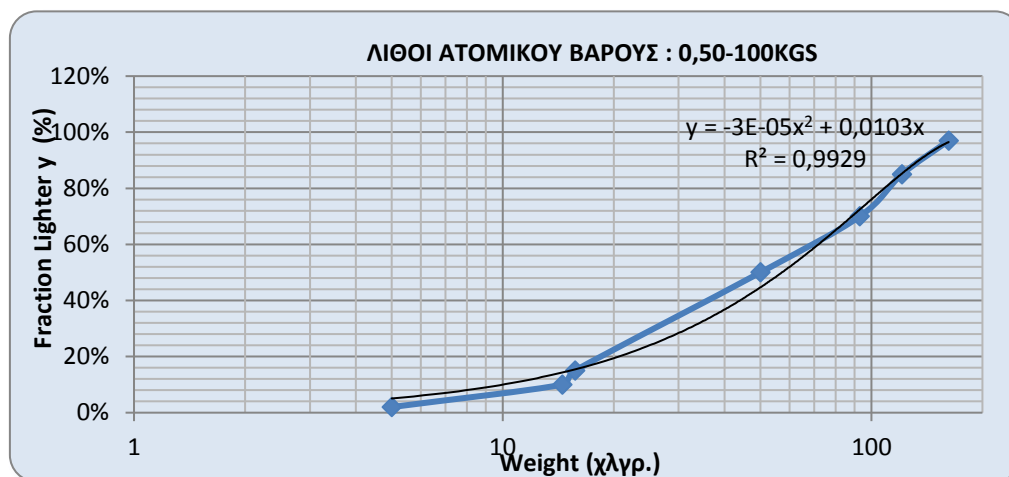
Σχήμα 3-6 Κοκκομετρική καμπύλη διαβάθμισης 0,5-100χγρ.
