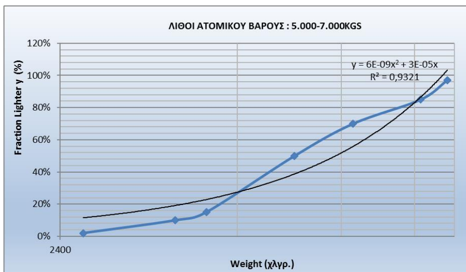
Σχήμα 3-3: Κοκκομετρική καμπύλη διαβάθμισης 5.000-7.000χγρ.
