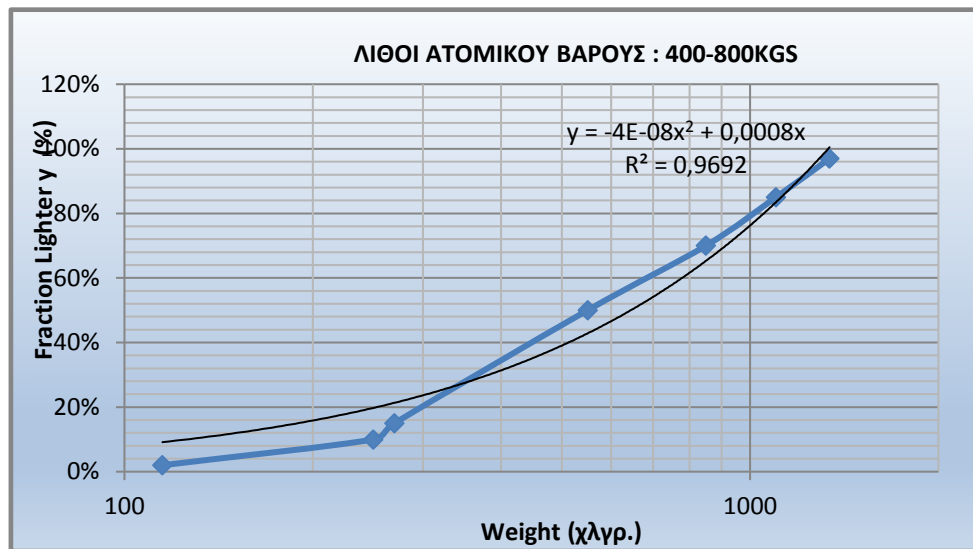
Σχήμα 3-1: Κοκκομετρική καμπύλη διαβάθμισης 400-700χγρ.
