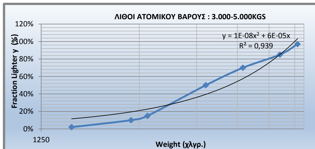
Σχήμα 3-2: Προδιαγραφές διαμόρφωσης καμπύλης υλικών, 3.000-5.000γρ.
